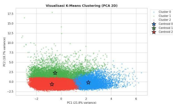
Gambar 5. Visualisasi K-Means Clustering (PCA 2D)
