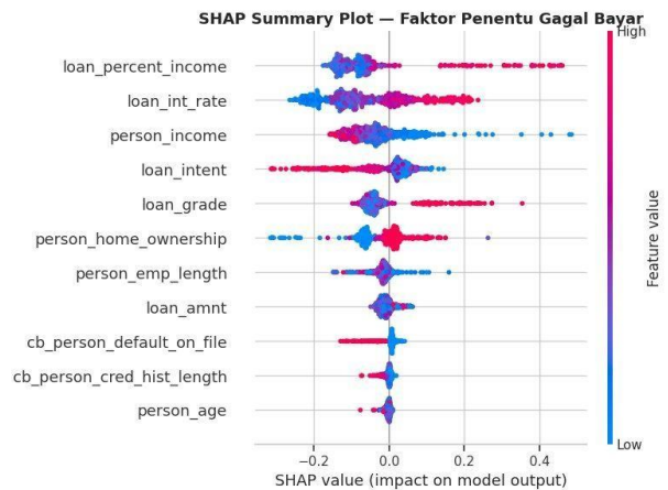
Gambar 3. SHAP Summary Plot — Faktor Penentu Gagal Bayar
